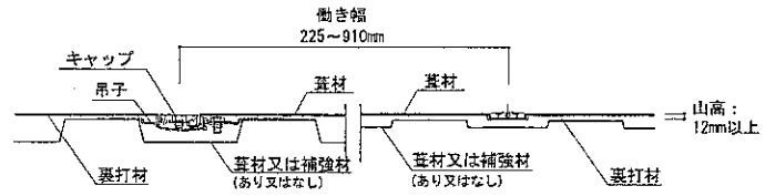
葺材断面図
