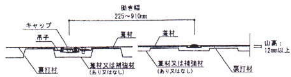
葺材断面図
