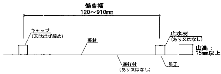
葺材断面 (代表的な仕様)
