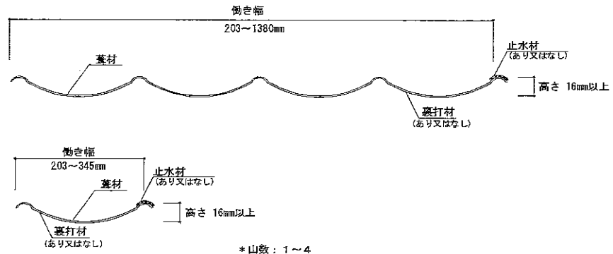
葦材断面 (代表的な仕様)
