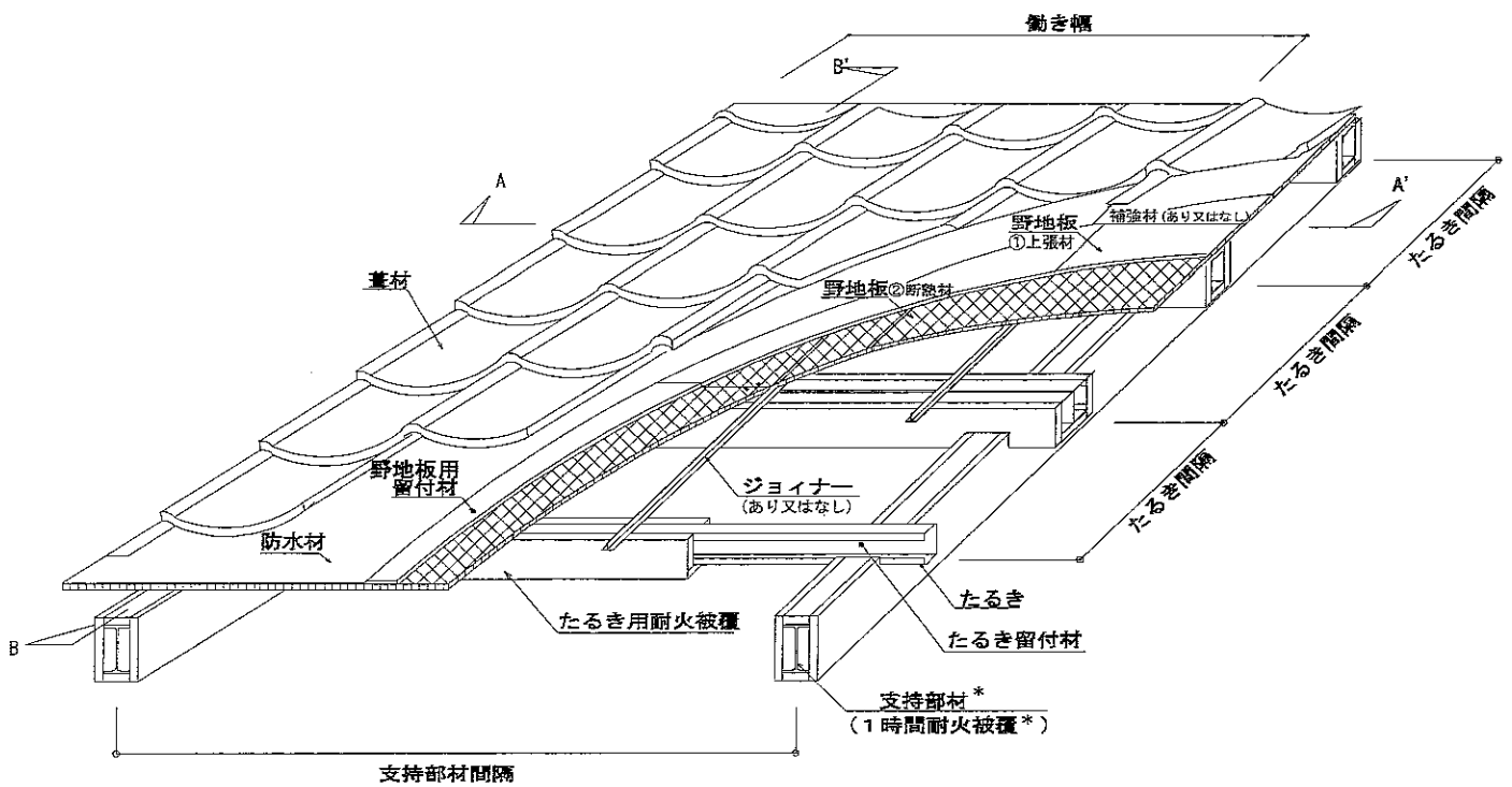
葦材断面 (代表的な仕様)
