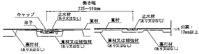
葺材断面図 (代表的な仕様)
